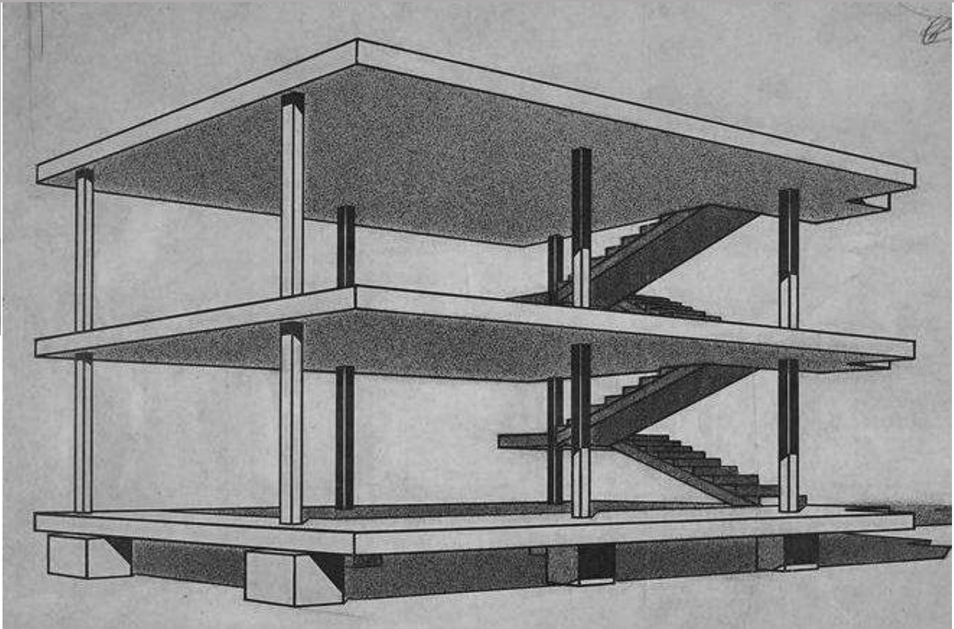
Système Dom-ino, croquis, 1914-15.
